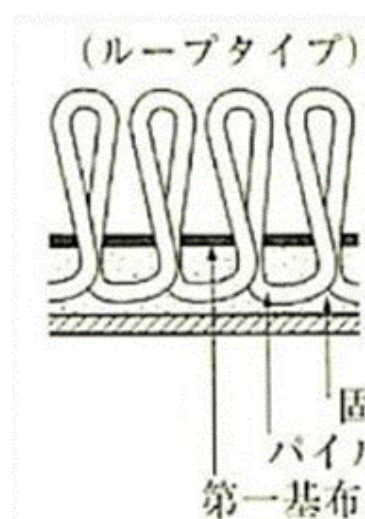
カーペットの構成断面図
